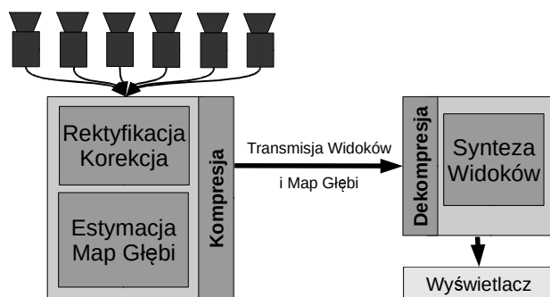
Rysunek 1. Schemat systemu telewizji swobodnego punktu widzenia
